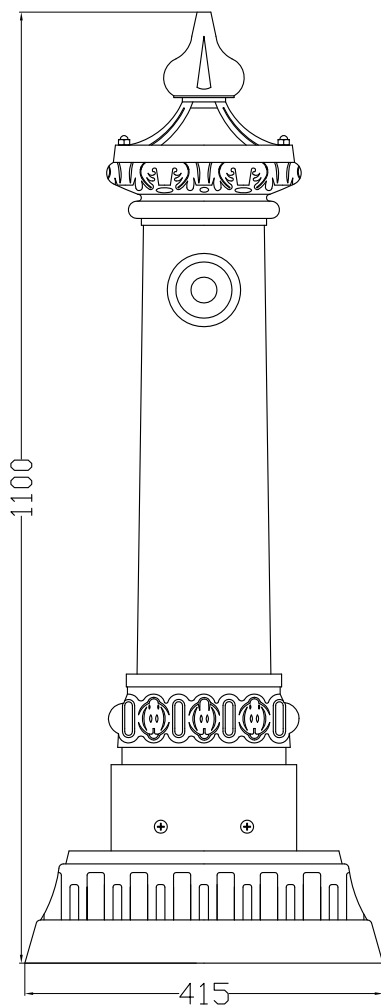
VISTA FRONTALE
