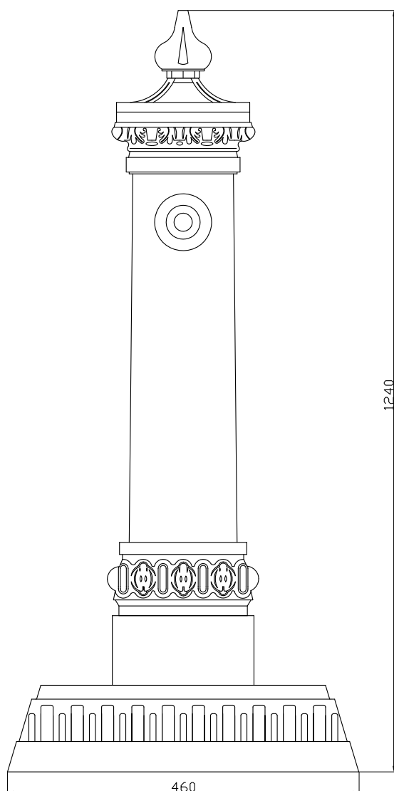
VISTA FRONTALE
