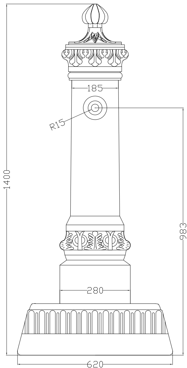
VISTA FRONTALE
