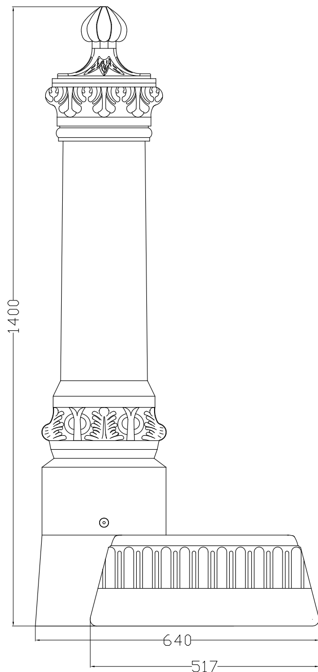
VISTA LATERALE
